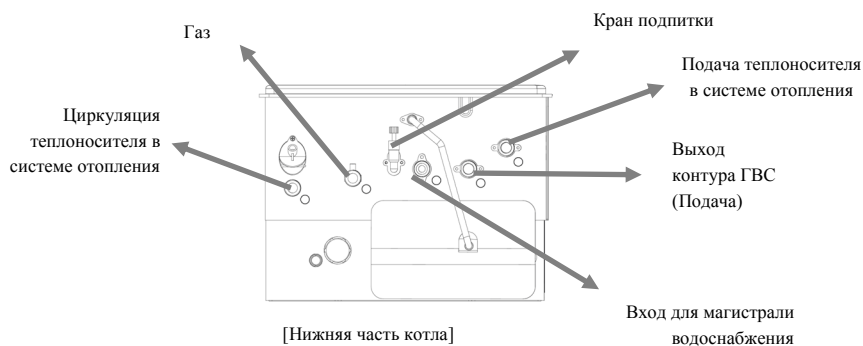
[Нижняя часть котла]
