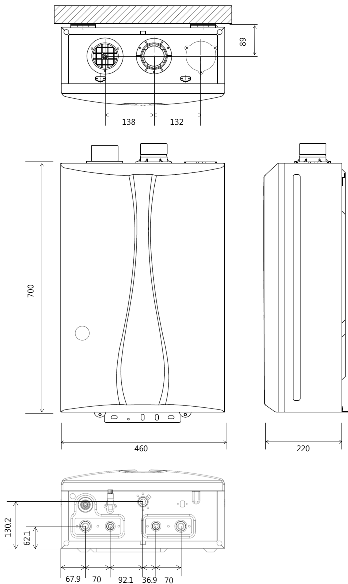
Модель A MAX 41
